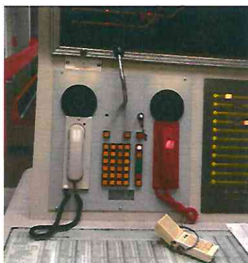
Platina de puntos fijos (señales de maniobra) en PML
