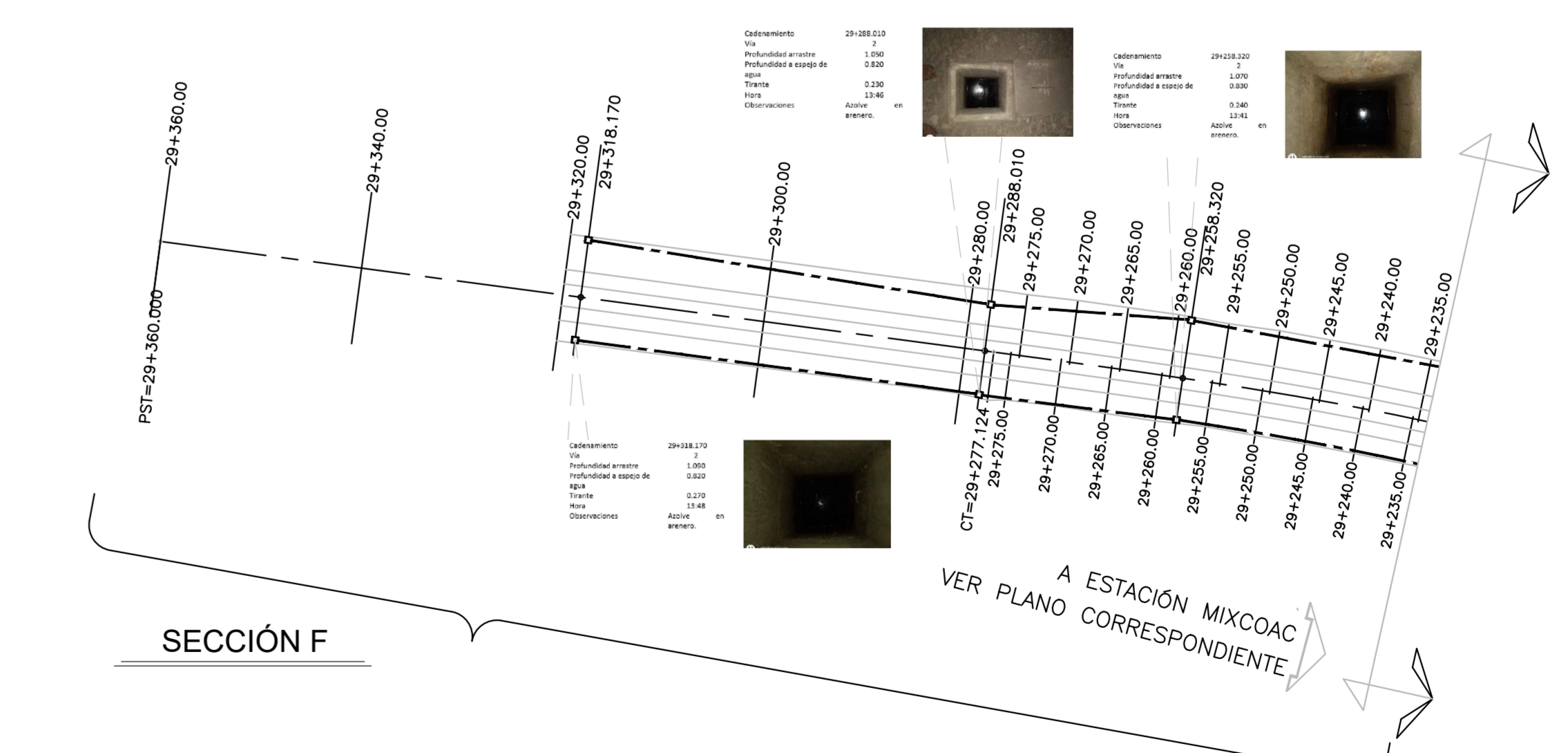
3 PLANTA DEL KM 29+235.00 AL KM 29+360.00 1 : 500
