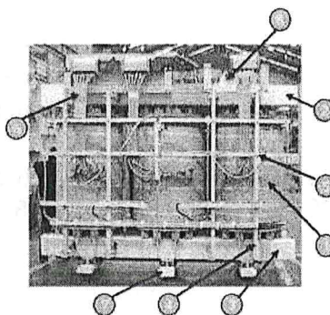
Imagen general de los devanados internos de un transformador
