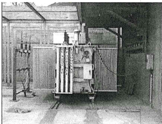
Transformador de potencia en Subestaciones de Rectificación de 23,000 volts.
