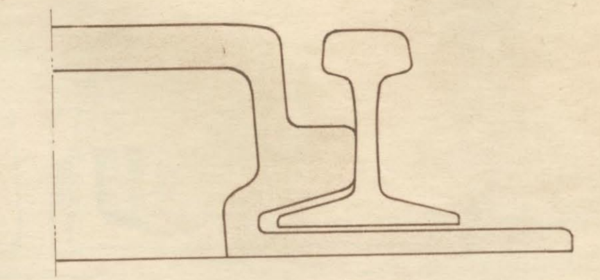
COUPE CC
