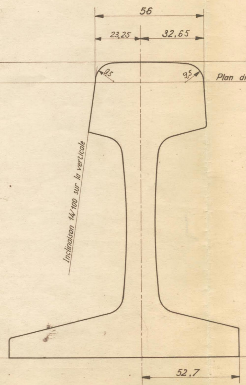
COUPE 4 à 2 569 de la P.R.A.
