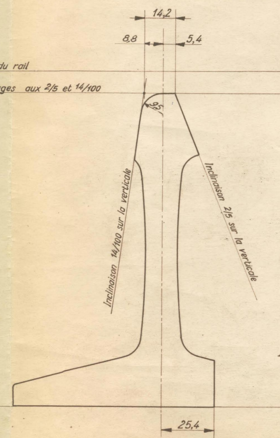
COUPE 2 P.M.A. à 800 de la P.R.A.
