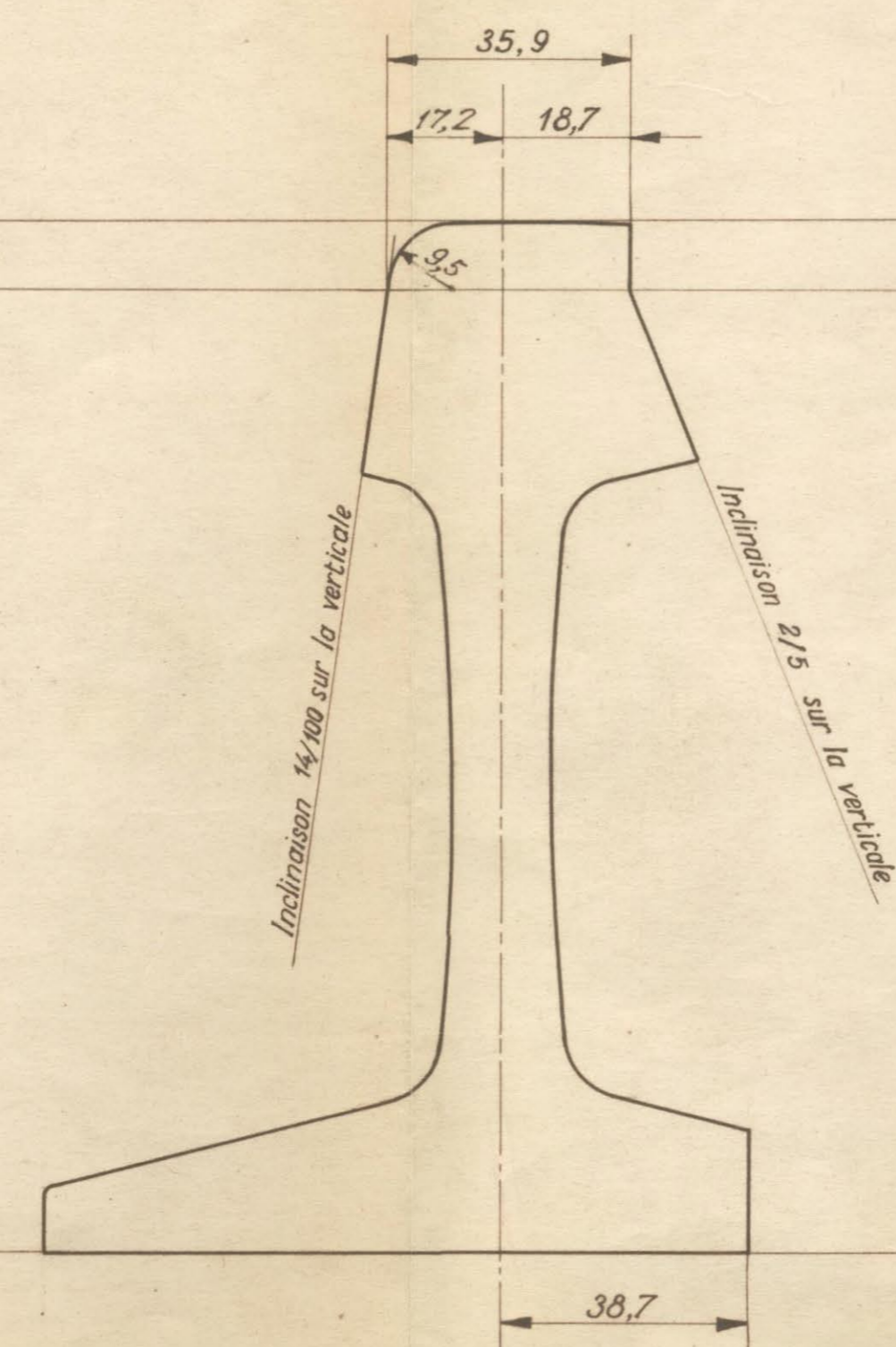
COUPE 3 à 1 824,5 de la P.R.A.
