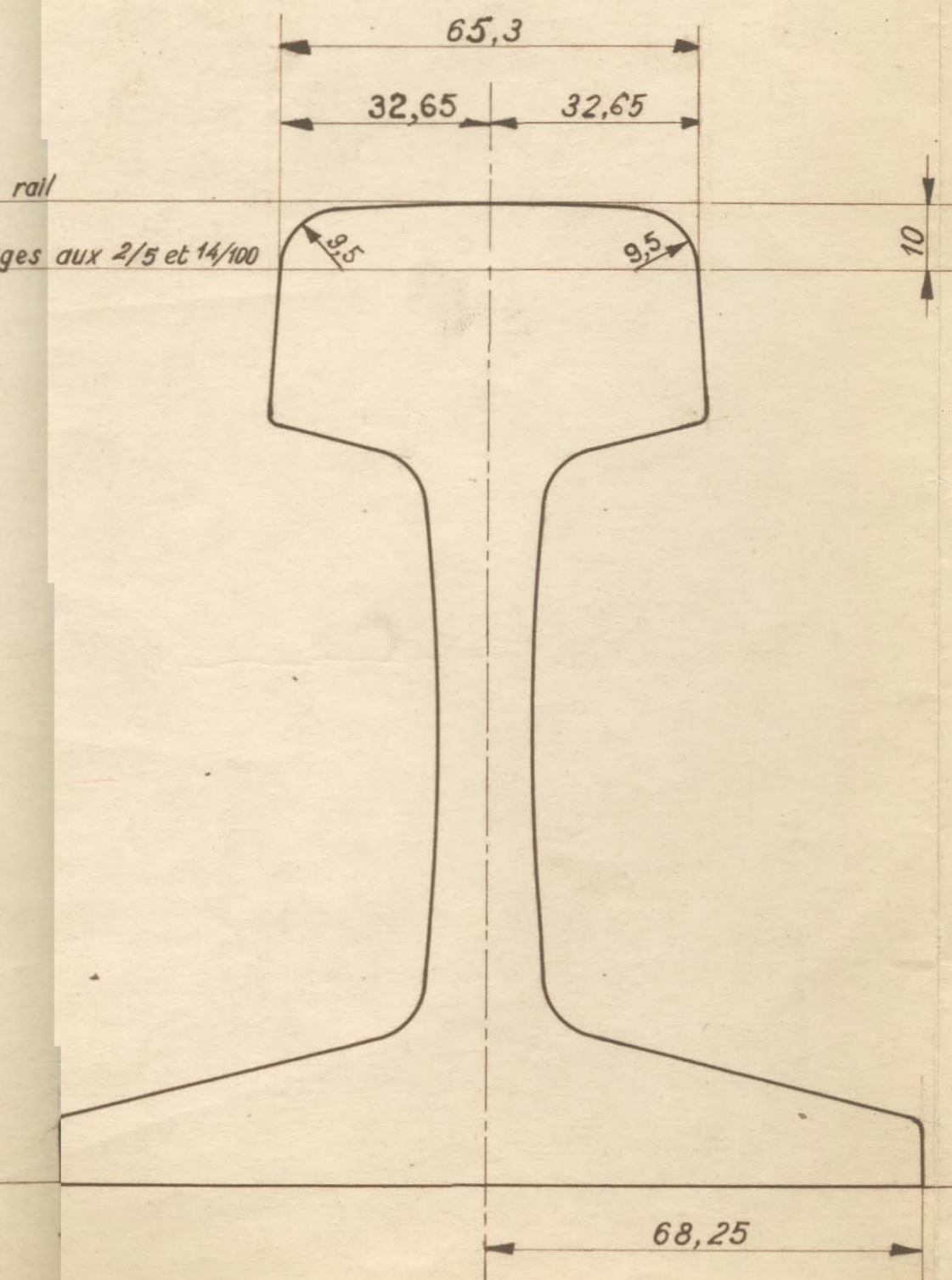
COUPE 5 à 3 720 de la P.R.A.
