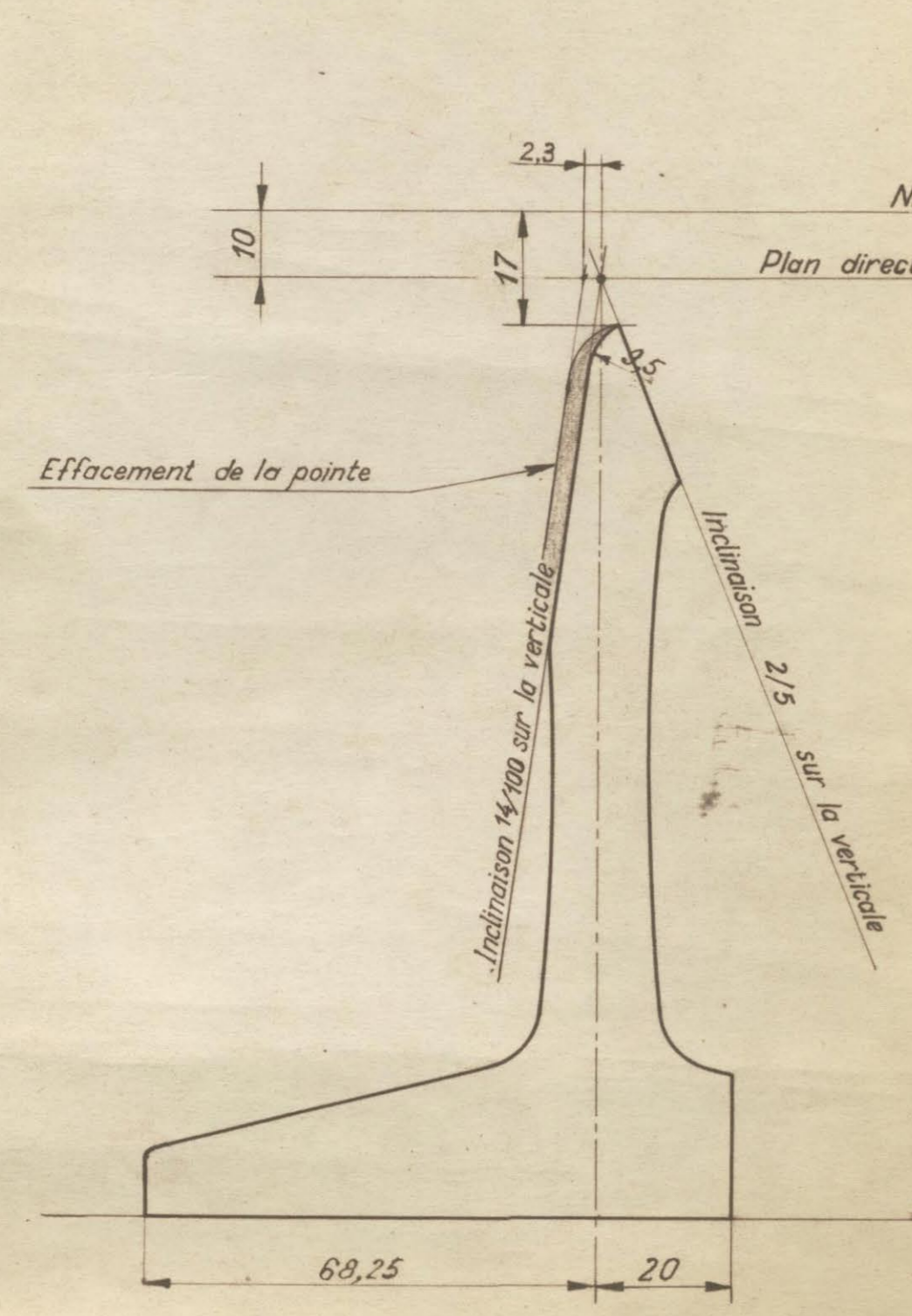
COUPE 1 à la P.R.A.
