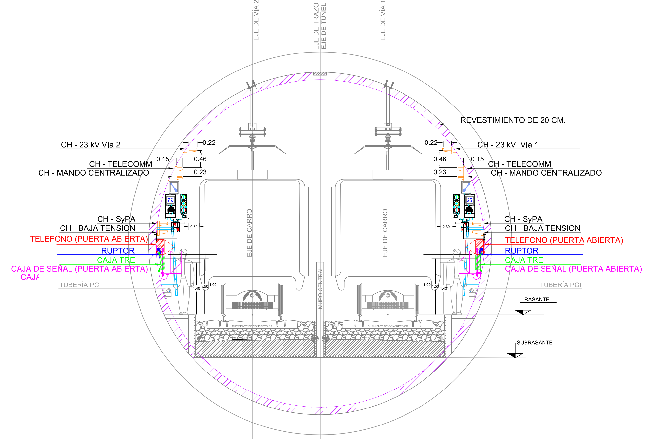
UBICACIÓN DE EQUIPOS ALSTOM EN SECCIÓN TIPO TUNEL CON REVESTIMIENTO DE 20 CM. (VER NOTA 3) COTAS EN MTS.
